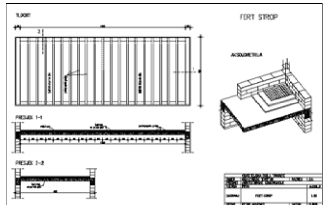
Tlocrt, presjek i aksonometrija fert stropa
