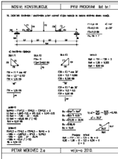
Nosive konstrukcije - proračun opterećenja na nosač
