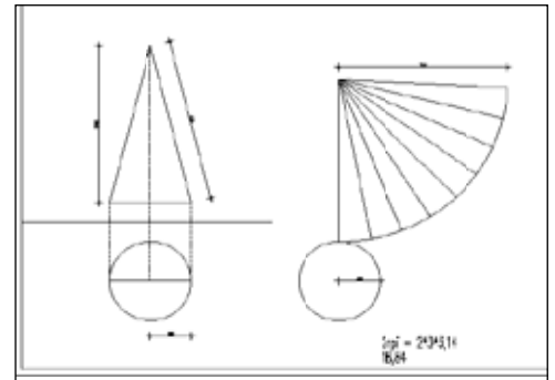
Tlocrt, nacrt i plašt stošca
