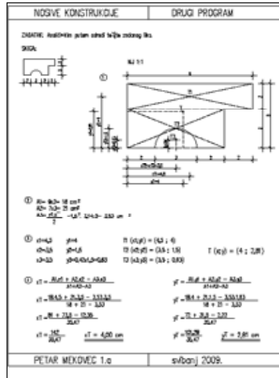
Analički proračun težišta tijela
