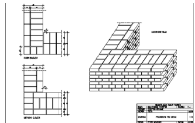
Aksonometrija i tlocrti pravokutnog veza opeke
